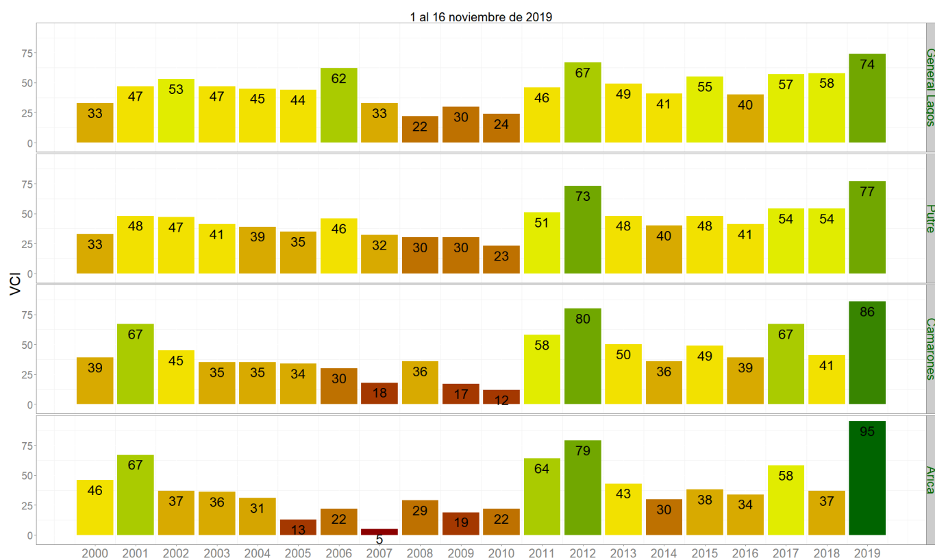
Figura 3. Valores del índice VCI para las 4 comunas con valores más bajos del índice del 1 al 16 noviembre 2019.
