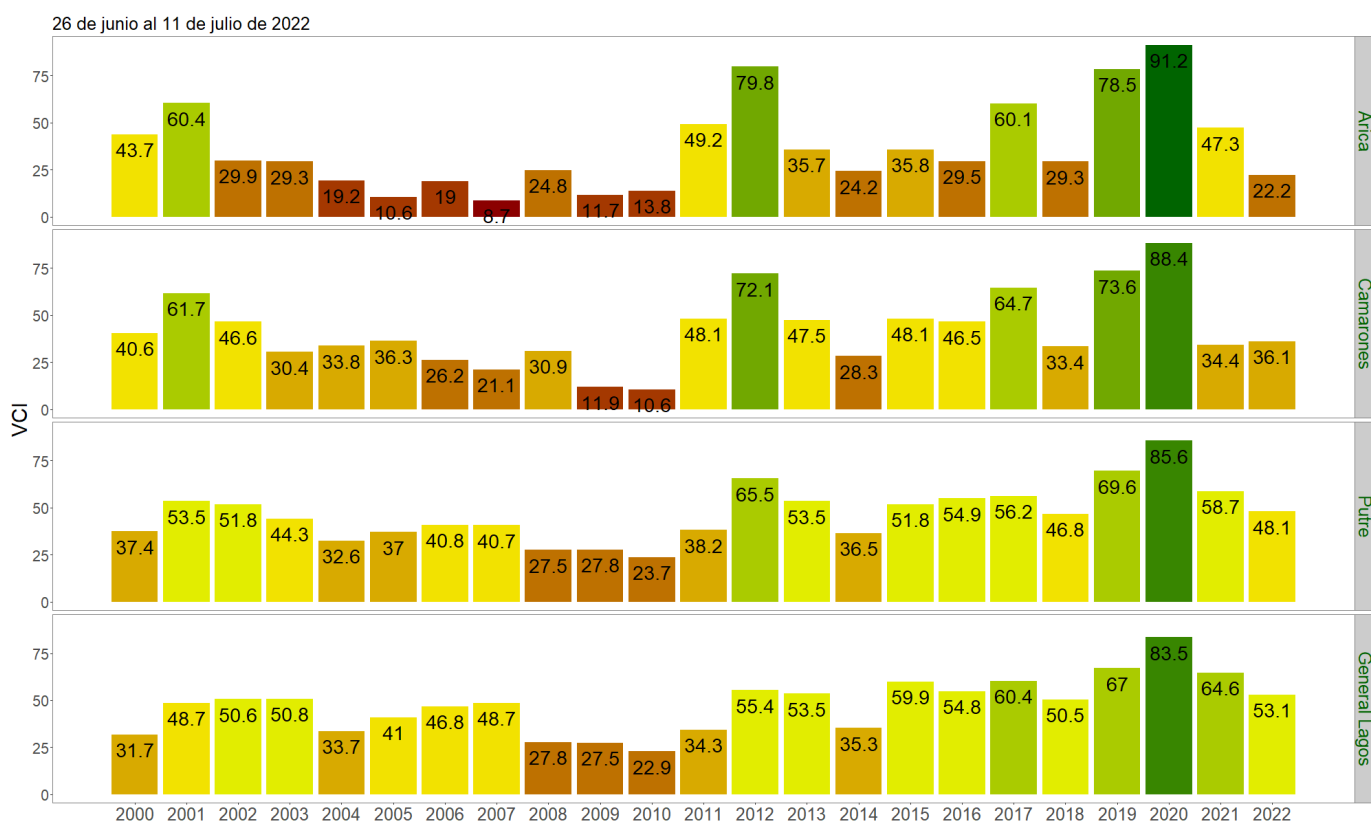
Figura 3. Valores del índice VCI para las 4 comunas con valores más bajos del índice del 26 de junio al 11 de julio de 2022.
