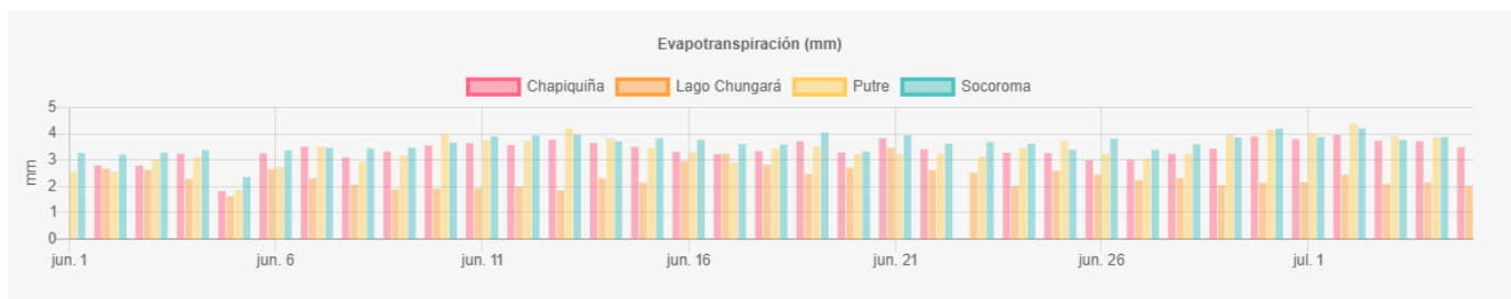
Figura 3. Evapotranspiración potencial (ETo) en mm/día, en las localidades de Chapiquiña, Lago Chungará, Putre y Socoroma (01 de junio, al 05 de julio 2022).
