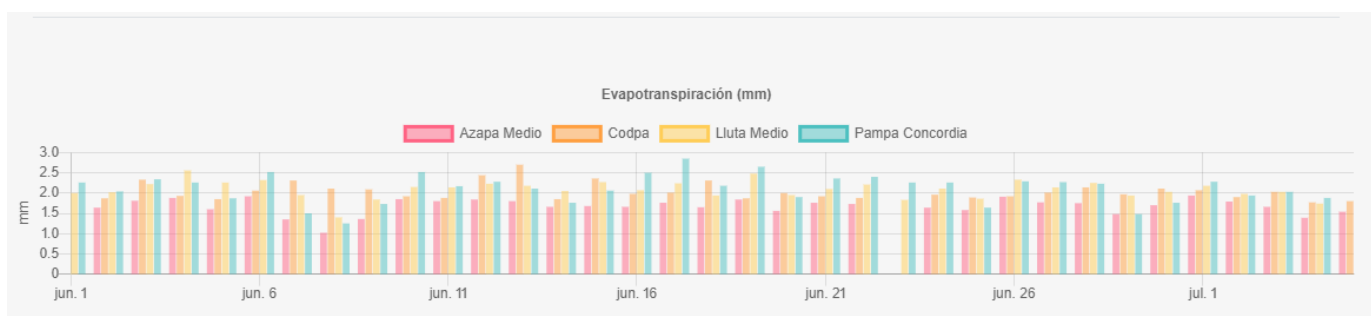
Figura 1.- Evapotranspiración potencial (ETo) en mm/día, en las localidades de Azapa Medio, Codpa, Lluta Medio y Pampa Concordia (01 de junio al 05 de julio 2022).
